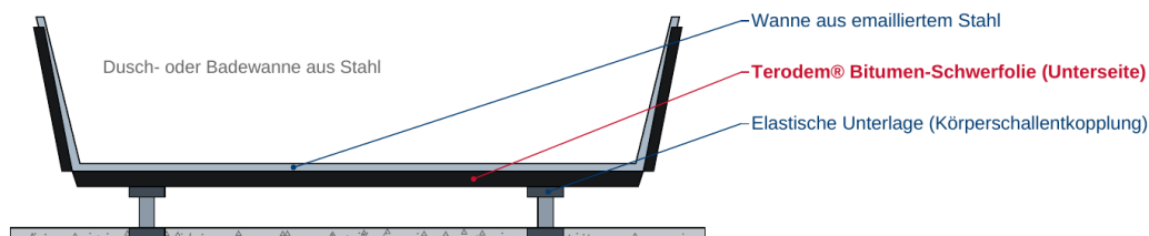
Querschnitt (schematisch)
