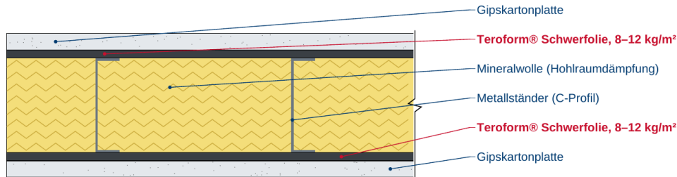
Horizontalschnitt (schematisch)
