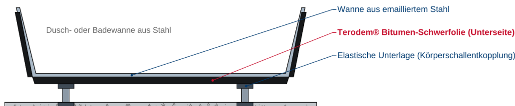
Querschnitt (schematisch)
