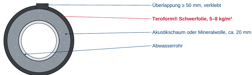
Querschnitt Rohrummantelung (schematisch)
