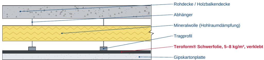
Vertikalschnitt (schematisch)
