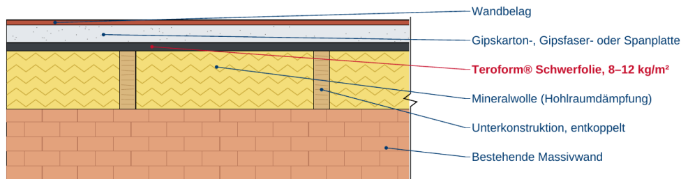
Horizontalschnitt (schematisch)
