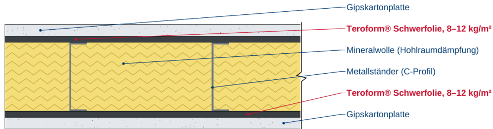
Horizontalschnitt (schematisch)
