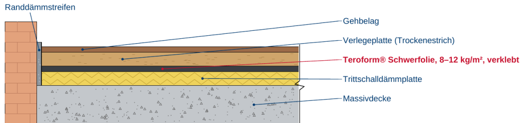
Vertikalschnitt (schematisch)
