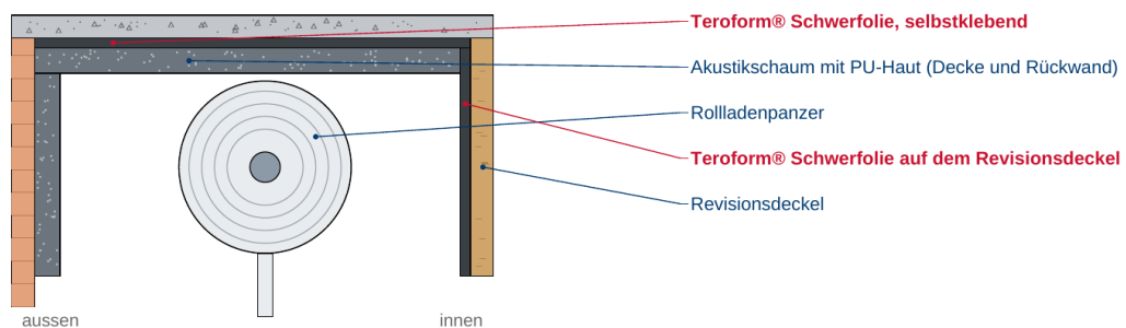
Querschnitt Rollladenkasten (schematisch)
