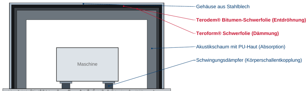
Schnitt durch eine Maschinenkapselung (schematisch)
