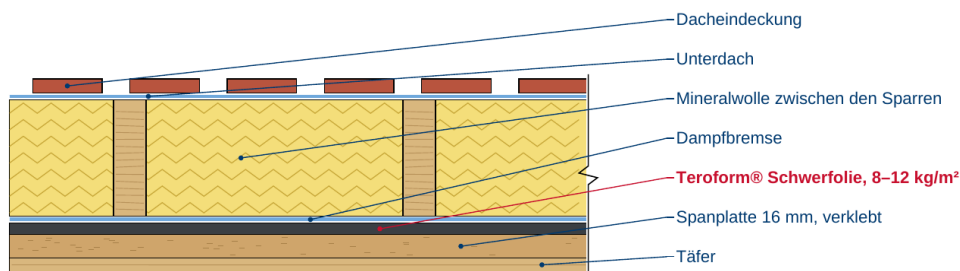
Schnitt senkrecht zur Dachfläche (schematisch)
