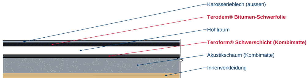
Schnitt durch Wand oder Boden (schematisch)
